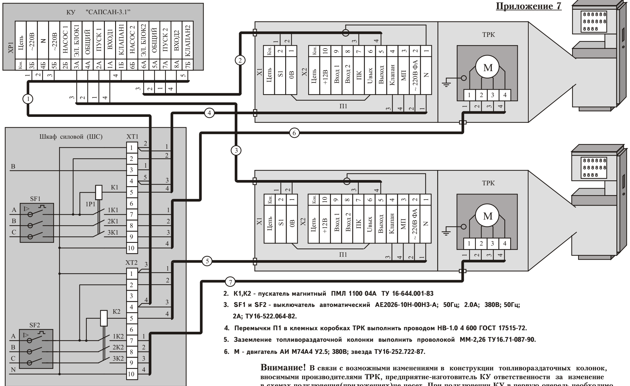
Схема соединения контроллера "САПСАН - 3.1" с ТРК "НАРА 28-5", "НАРА 28-16"
